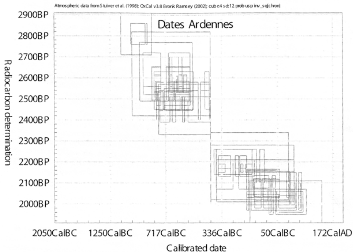
Fig. 2 : Graphique avec les datations ^{14}\text{C} calibrées pour les Ardennes, au sud du massif Ardennais. Les blocs représentent la fourchette de datation (largeur) et la probabilité (hauteur) à deux sigma, à l'intérieur, les blocs plus petits indiquent les datations à 1 sigma.
